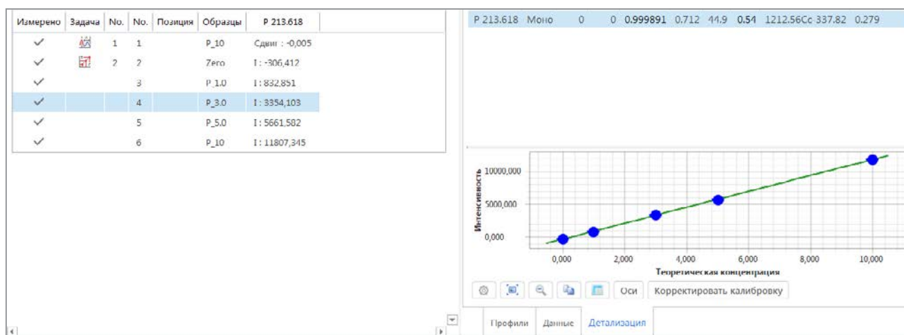
Рис. 1. График градуировки
