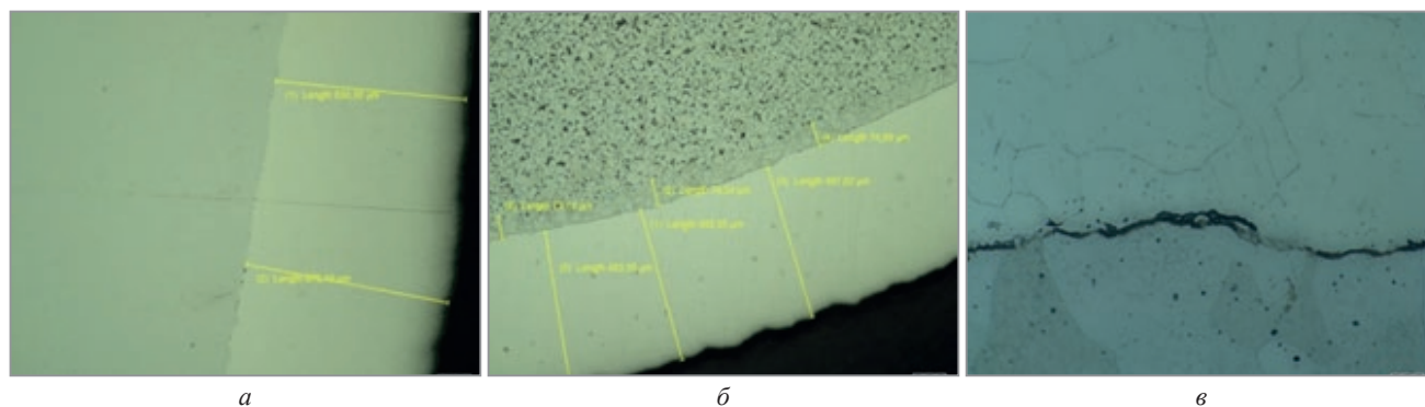
Рис. 2. Полированный образец (а). \times 100 ; травление в реактиве «Nitall» (б). \times 100 ; выявленные границы зерен нержавеющей аустенитной стали (в). \times 1000
