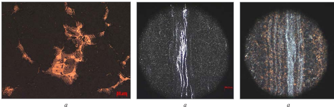
Рис. 2. Карбидная ликвация в структуре стали марки 100Cr6, травление в 10%-ном растворе азотной кислоты в спирте: а – карбидная ликвация в осевой зоне НЗЛ. x200; б – карбидная ликвация и карбидная полосчатость в осевой зоне горячекатаного прутка. x100
