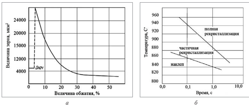
Рис. 4. Влияние деформационных и температурных параметров прокатки на структуру проката из подшипниковых сталей: а – зависимость размера зерна от степени деформации; б – влияние температуры конца прокатки на рекристаллизацию
