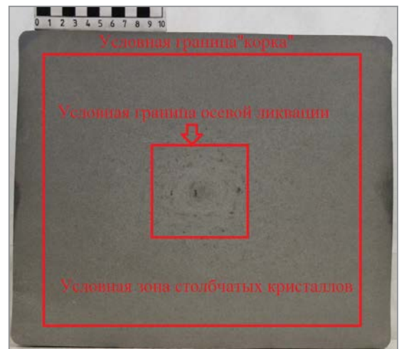
Рис. 1. Внешний вид поперечного сечения темплет
