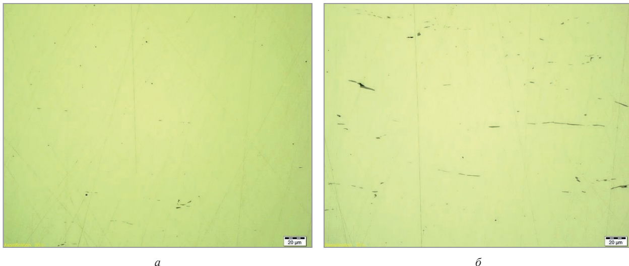
Максимальные размеры неметаллических включений в виде сульфидов и оксидов в плавках: а – опытные; б – сравнительные. \times 200
